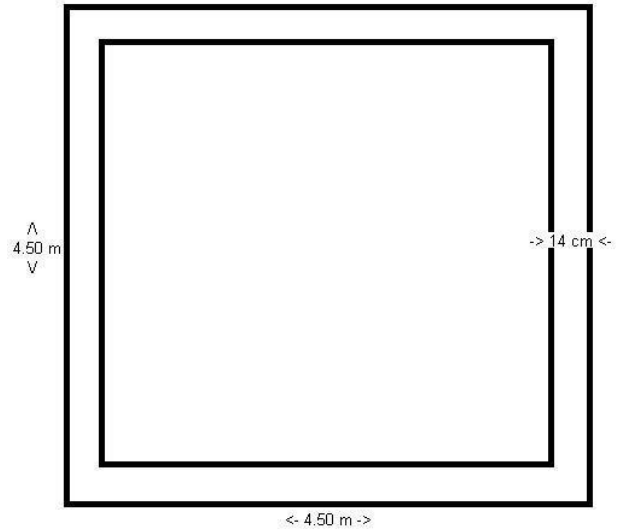
Bovenaanzicht spant
